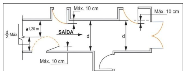
Figura 2: Abertura das portas no sentido de saída
