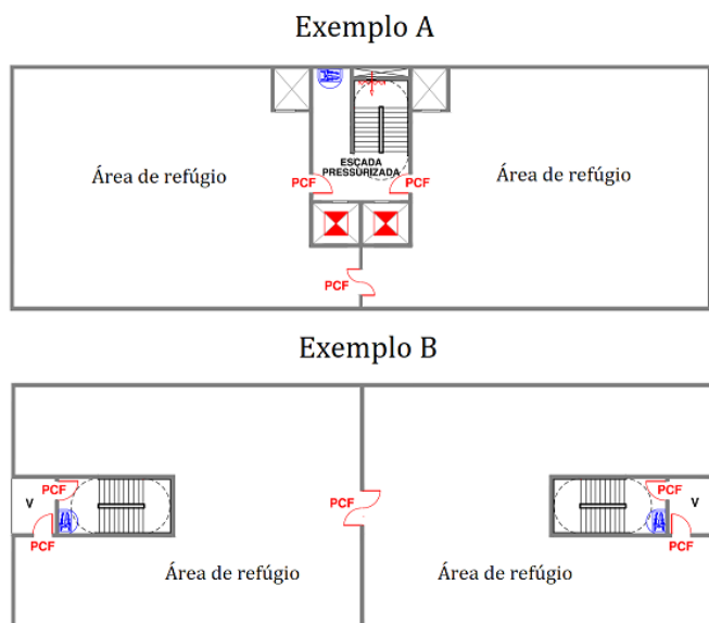
Figura 25: Exemplos esquemáticos de áreas de refúgio (ilustrativo).
