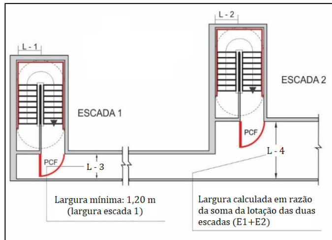
Figura 26: Dimensionamento de corredores de descarga.
