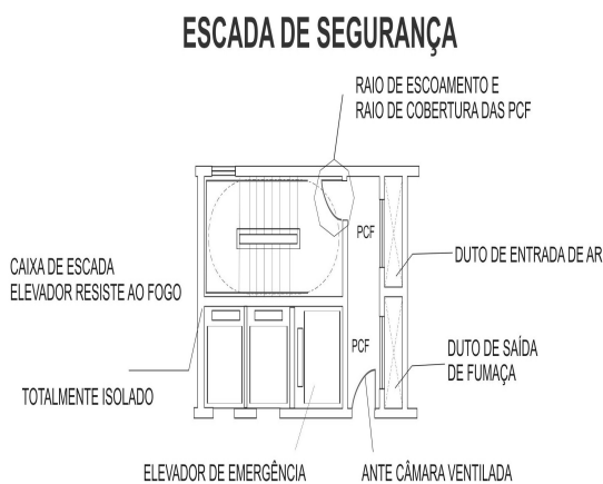
Figura 51 - Escada e elevador à prova de fumaça
