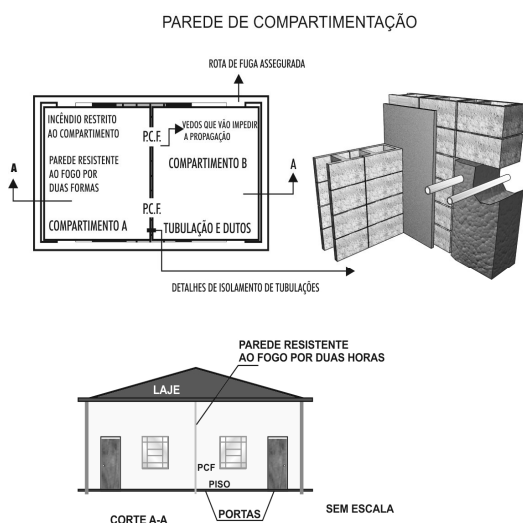
Figura 32 - Detalhes de parede de compartimentação
