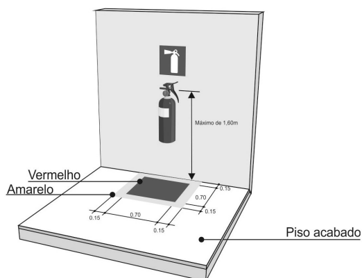
Figura 62 - Detalhe de instalação de extintores em áreas sujeitas à obstrução
