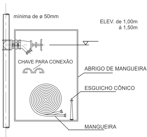
Figura 63 - Detalhe de hidrante
