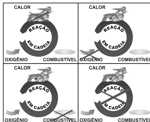
Figura 19 - Formas de extinção do fogo
