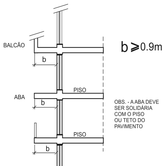
Figura 34 - Compartimentação por aba horizontal ou balcão
