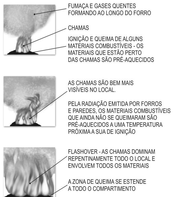
Figura 38 - Evolução da propagação nos materiais
