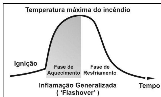
Figura 20 - Curva temperatura - tempo de um incêndio
