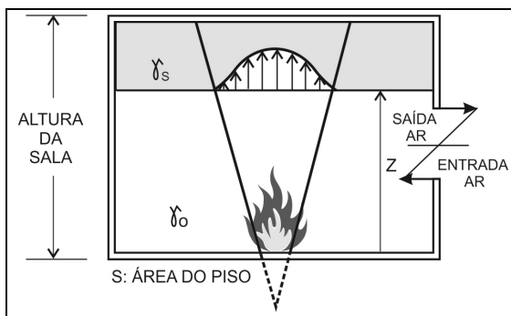
Figura 27 - Processo de formação de gases e fluxo básico de ar
