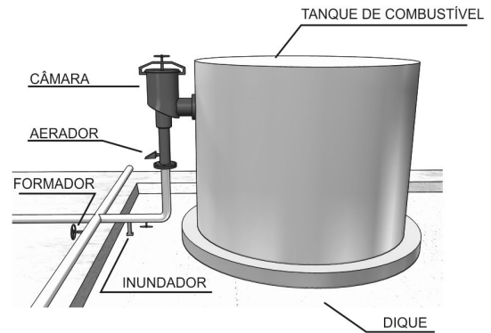
Figura 72 - Detalhe de câmara de espuma
