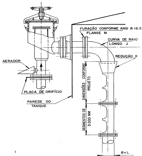
Figura 70 - Sistema fixo de espuma
