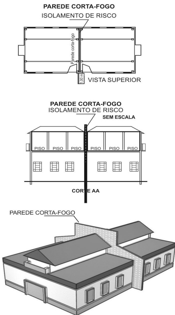
Figura 31 - Isolamento obtido por parede corta-fogo
