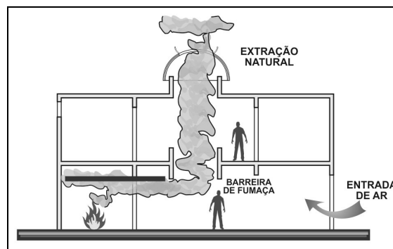
Figura 28 - Extração de fumaça de átrios
