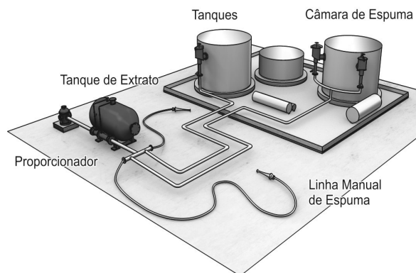
Figura 71 - Sistema semifixo
