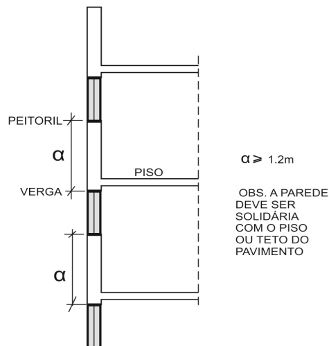
Figura 33 - Distância de afastamento entre verga e peitoril
