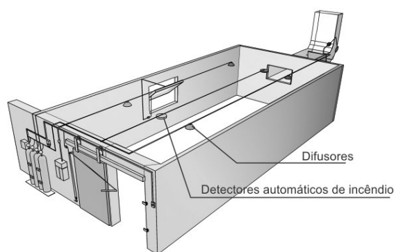
Figura 73 - Sistema de CO 2
