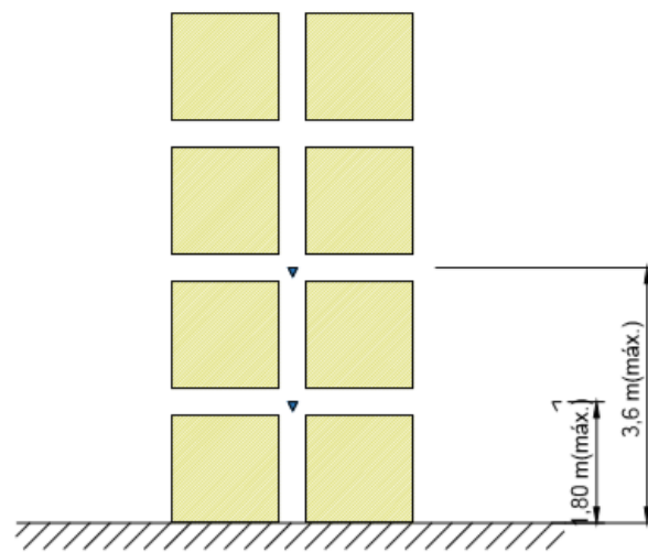
Elevação frontal
