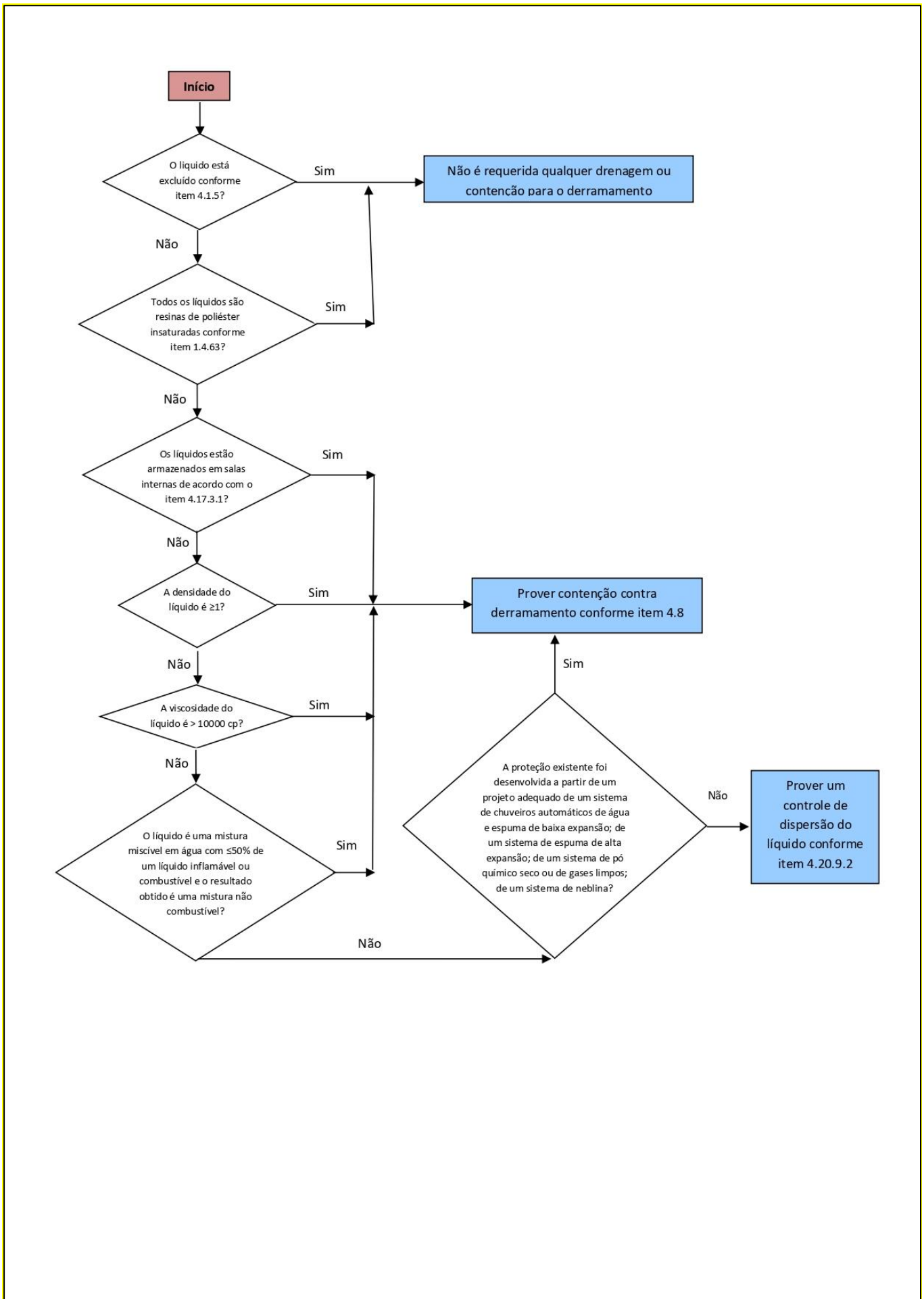
Figura 4.5 – Contenção de derramamentos e controle de dispersão de líquidos em áreas de armazenamento protegido
