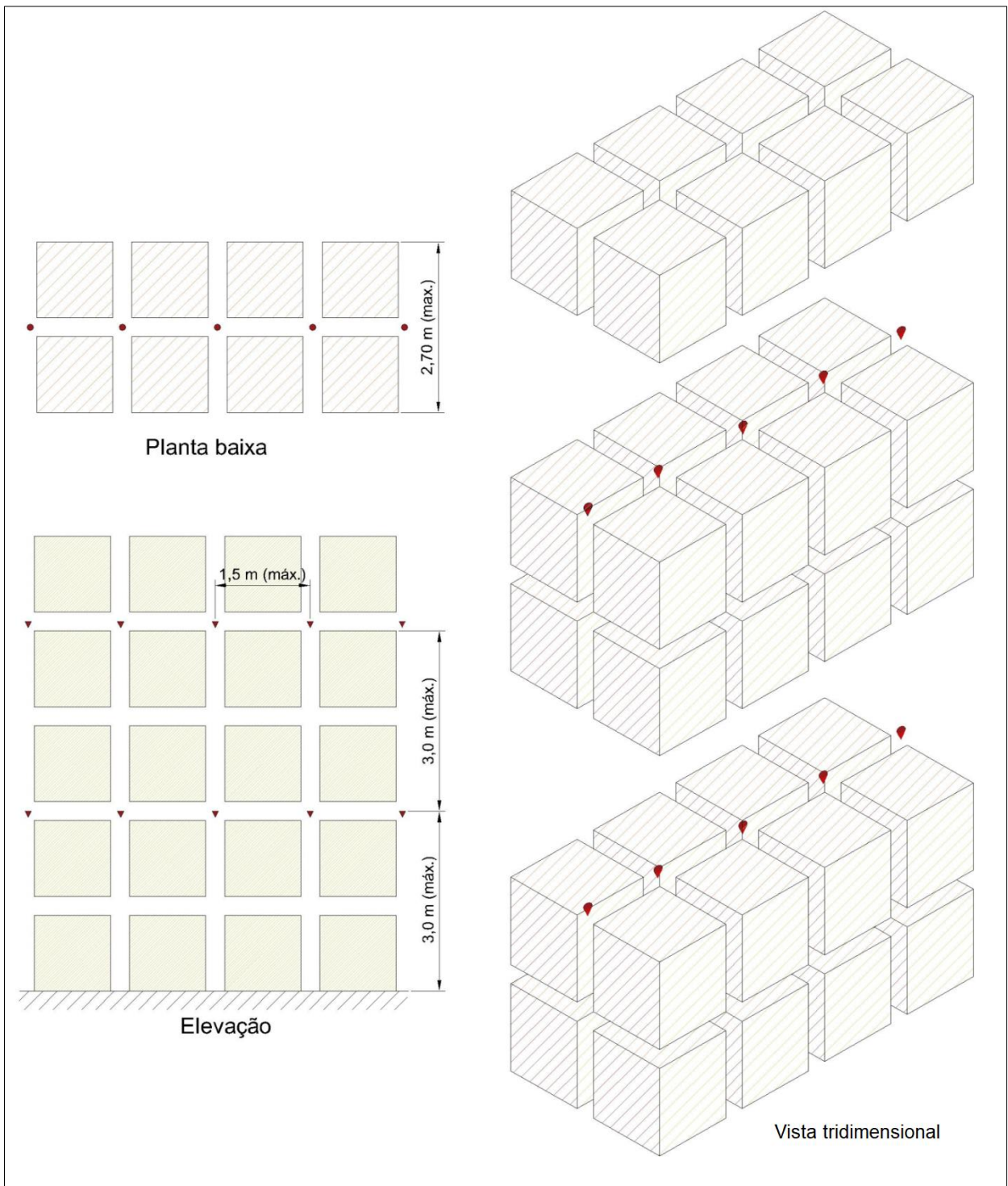
Figura 4.17: Leiaute de chuveiros automáticos para estrutura-suporte de fileira dupla – Leiaute “1” - Opção # 2.
