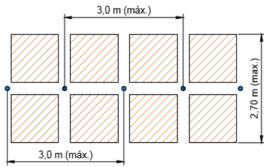
Planta baixa
