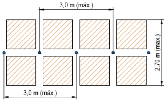
Planta baixa
