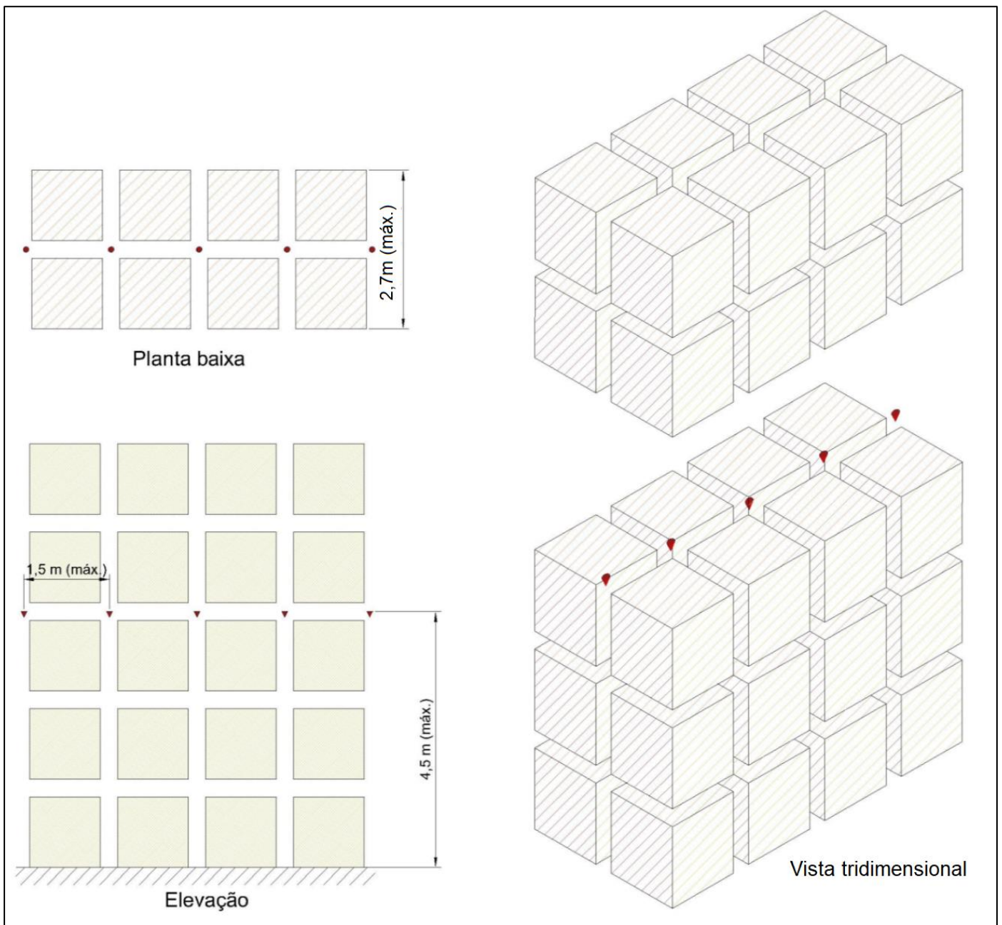
Figura 4.19: Leiaute de chuveiros automáticos para estrutura-suporte de fileira dupla – Leiaute "H" - Opção # 2.
