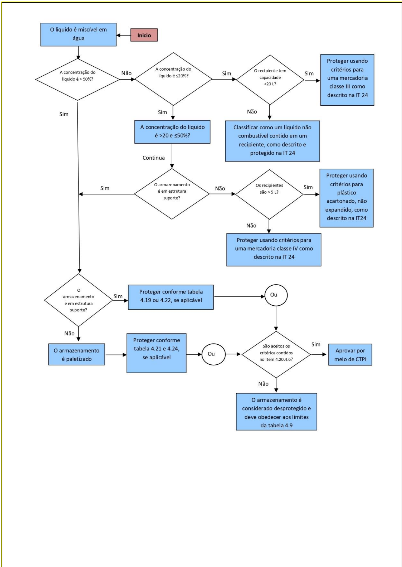
Figura 4.4 – Árvore de decisão para o critério de proteção contra incêndio para líquidos inflamáveis e combustíveis miscíveis em água contidos em recipientes não metálicos
