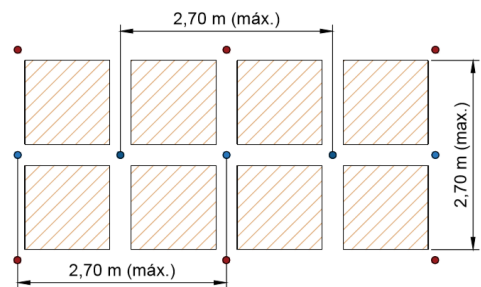
Planta baixa
