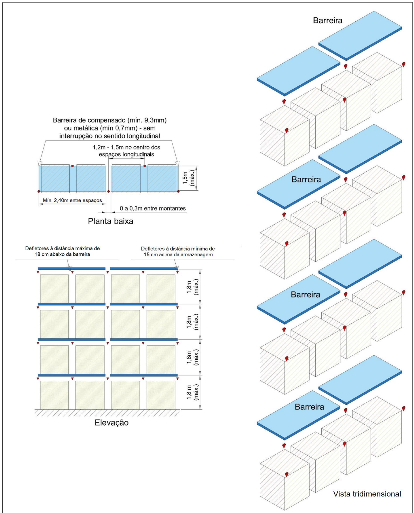
Nota: ▼ Chuveiros automáticos de níveis intermediários, chuveiros-spray, resposta rápida (QR), K 115. Figura 4.10: Leiaute de chuveiros automáticos para estrutura-suporte de fileira única – Esquema de projeto “B” – Chuveiros voltados para a estrutura.
