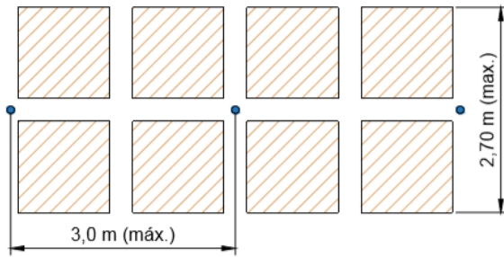
Planta baixa
