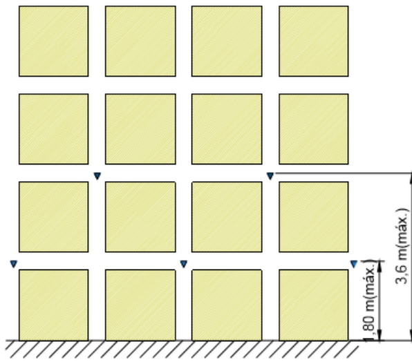
Elevação lateral
