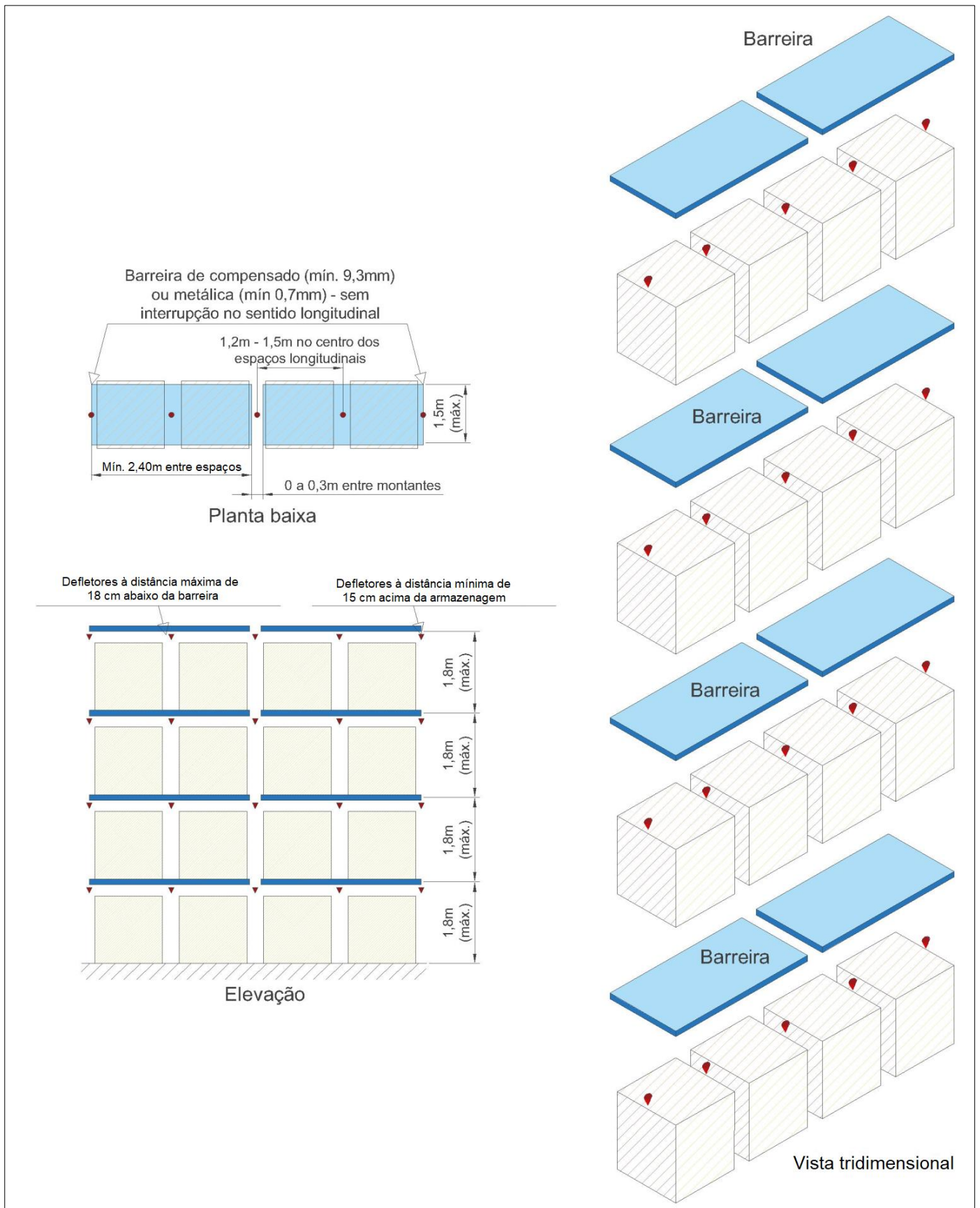
Nota: ▼ Chuveiros automáticos de níveis intermediários, chuveiros-spray, resposta rápida (QR), K 115. Figura 4.9: Leiaute de chuveiros automáticos para estrutura-suporte de fileira única Esquema de projeto "B" – Chuveiros no centro da estrutura.
