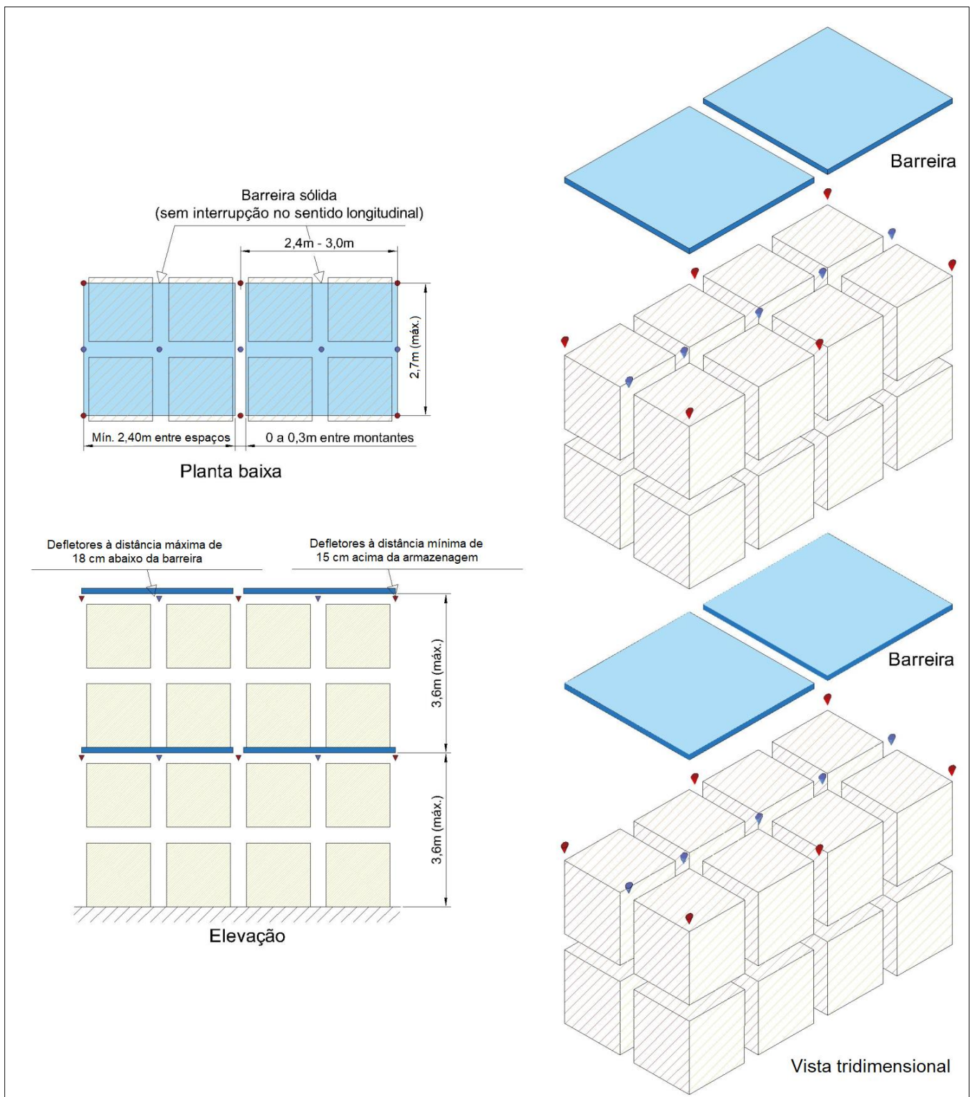
Figura 4.7: Leiaute de chuveiros automáticos para uma estrutura-suporte de fileira dupla – Esquema de projeto “A”
