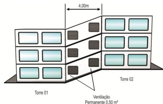
Figura 12 – Abertura lateral na escada
