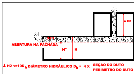
Figura 17 - Diâmetro hidráulico
